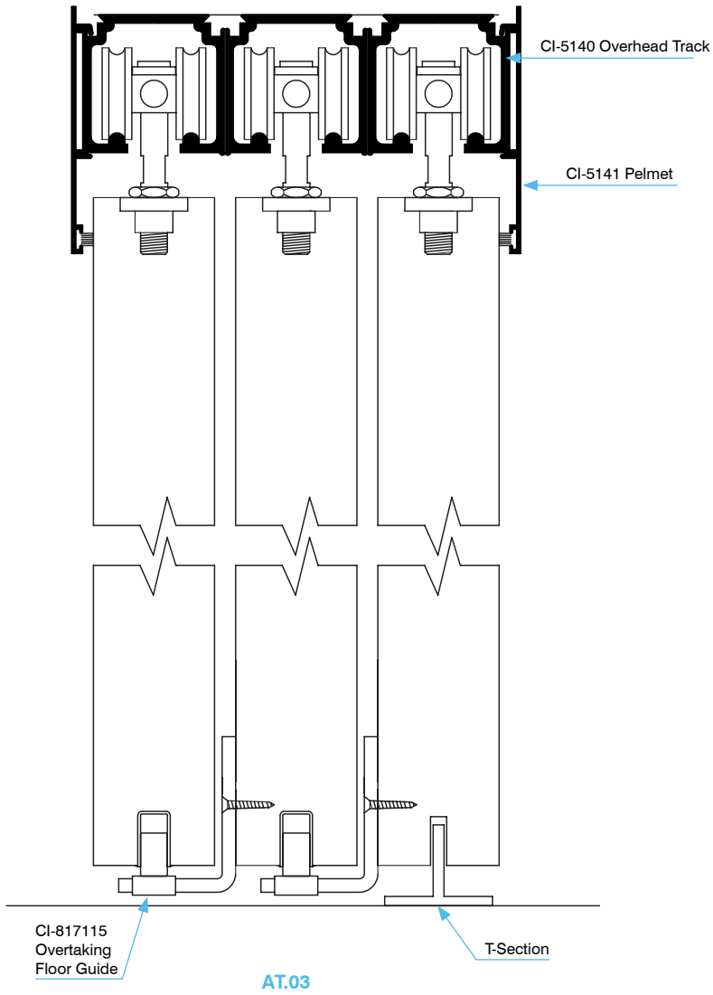
ELEVATION
